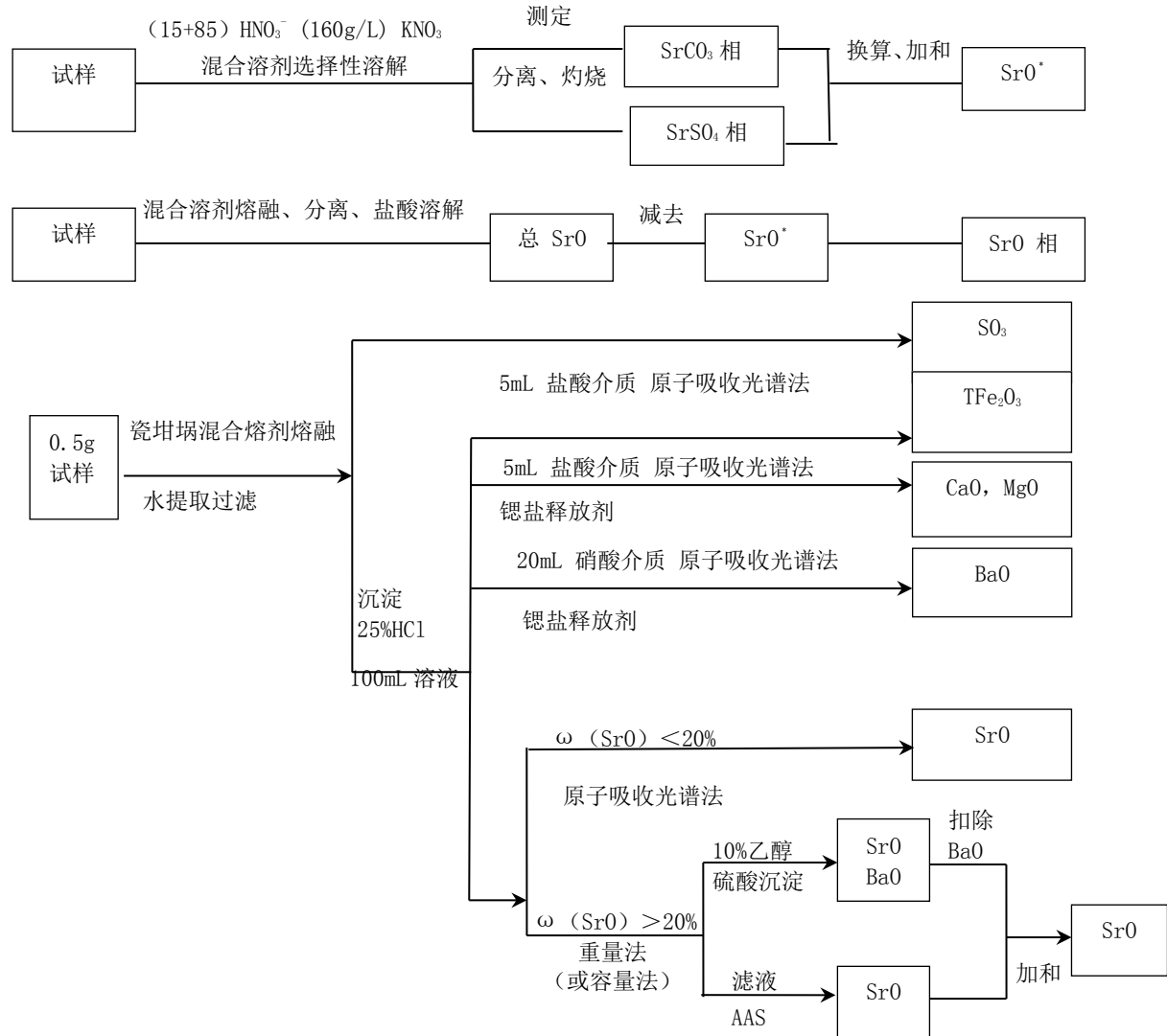
图 B. 1 天青石矿物质量分数测定流程图
